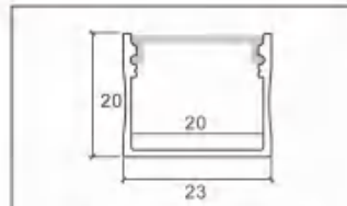
型号: 2320M/21页
