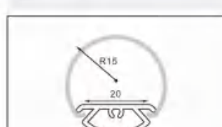
型号: Ø30/42页
