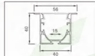
型号: 4040A/25页
