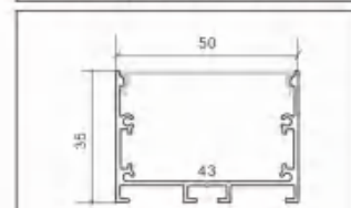
型号: 5035M/27页
