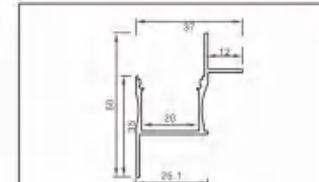
型号: 102/55页
