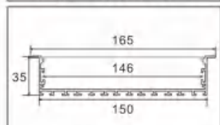
型号: 15035A/37页
