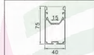
型号: 4075M/26页
