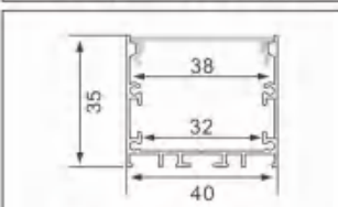
型号: 4035M/25页
