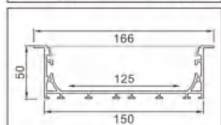
型号: 15050A/37页
