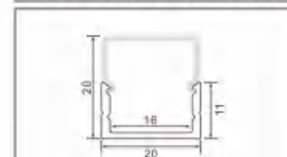
型号: 2011/19页
