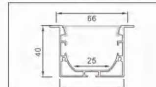
型号: 5040A/28页
