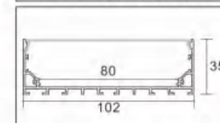
型号: 10235M/35页
