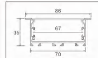
型号: 7035A/30页
