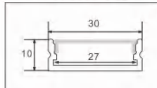
型号: 3010M/21页
