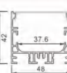
型号: 4842M/02页
