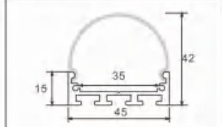
型号: 4542圆/42页
