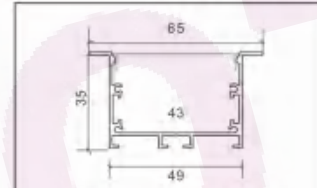
型号: 5035A/27页
