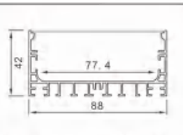
型号: 8842M/06页
