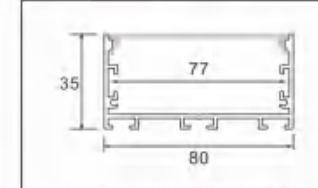
型号: 8035M/32页
