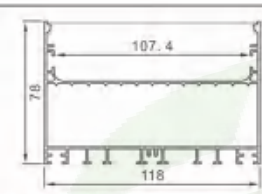
型号: 11878M/08页
