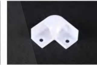
PC转接头:601转角 内空尺寸:15.8*15.8MM
