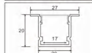
型号: 2020A/20页
