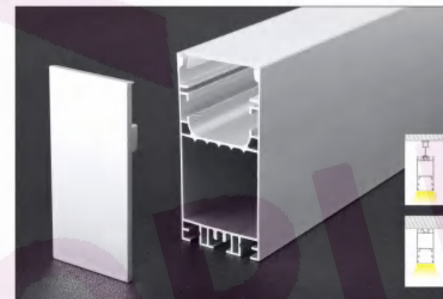
塑料堵头 plastic end cap 金属卡子 spring clip 吊线 suspended wire
