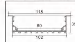
型号: 10235A/35页
