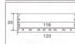
型号: 12035M/35页
