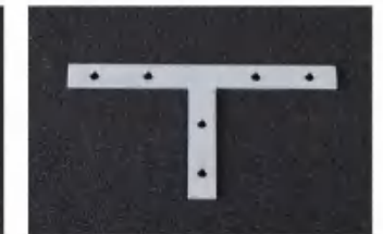
T字连接片 100mm*10mm*2mm 内六角M4螺丝
