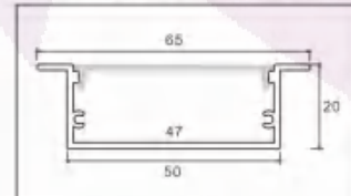
型号: 5020A/26页
