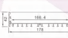
型号: 17842M/09页
