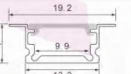
型号: 510A/12页
