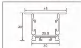
型号: 3030A/22页
