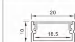
型号: 2010M/18页
