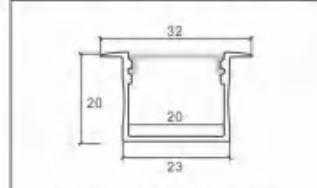
型号: 2320A/21页
