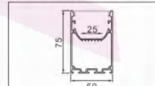
型号: 5075M/29页
