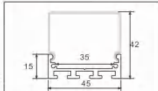
型号: 4542方/42页
