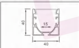
型号: 4040M/25页
