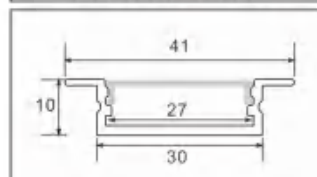
型号: 3010A/21页
