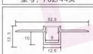
型号: 639新款/45页
