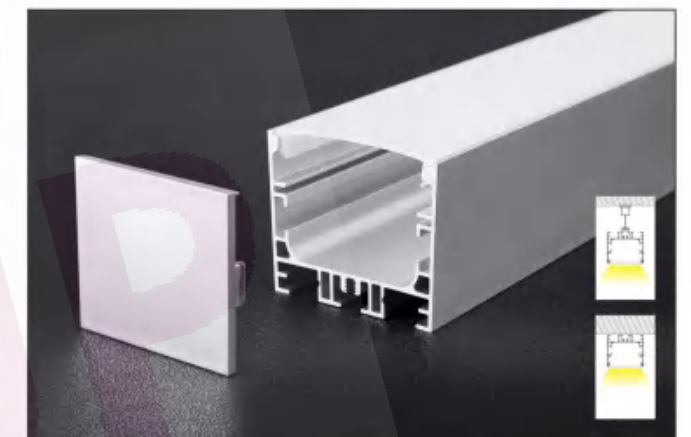
塑料堵头 plastic end cap 金属卡子 spring clip
