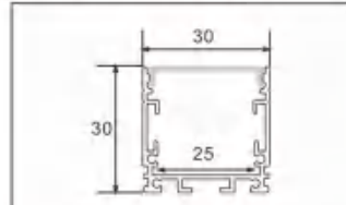
型号: 3030M/22页
