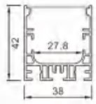
型号: 3842M/02页
